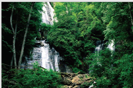
Rừng (cây xanh) là bể hấp thụ và bể chứa cacbon
