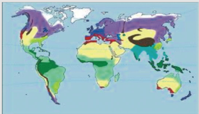
Bản đồ phân vùng khí hậu của Việt Nam (Nguyễn Đức Ngữ - ảnh trái) và của thế giới (my.opera.com-ảnh phải)
