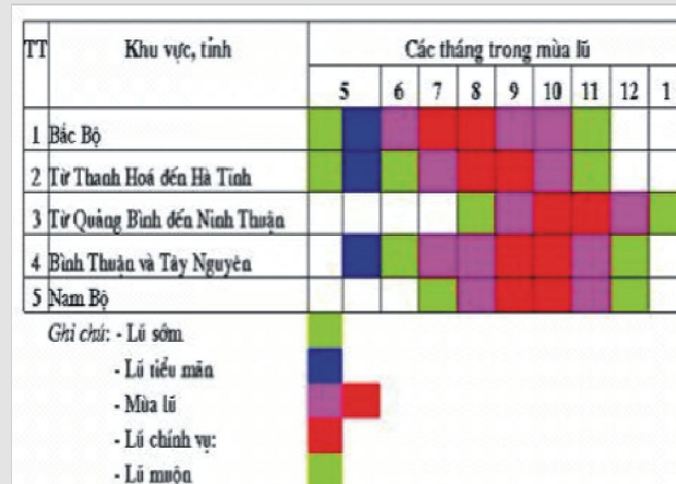
Mùa lũ ở các khu vực (Trung tâm Khí tượng Thủy văn Quốc gia, 2011)
