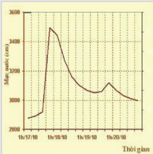
Đường quá trình lũ tại trạm Sơn Giang năm 1999
