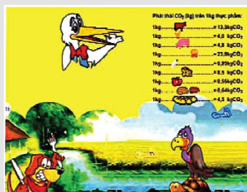
Phát thải KNK (Tamnhin.net, greenbiz.vn)
