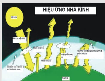
Hiệu ứng nhà kính nhà kính trồng cây (muchapedia.com) (muchapedia.com)
