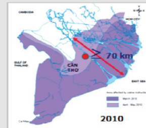
Ở ĐBSCL mặn đã vào sâu tới 70 km
